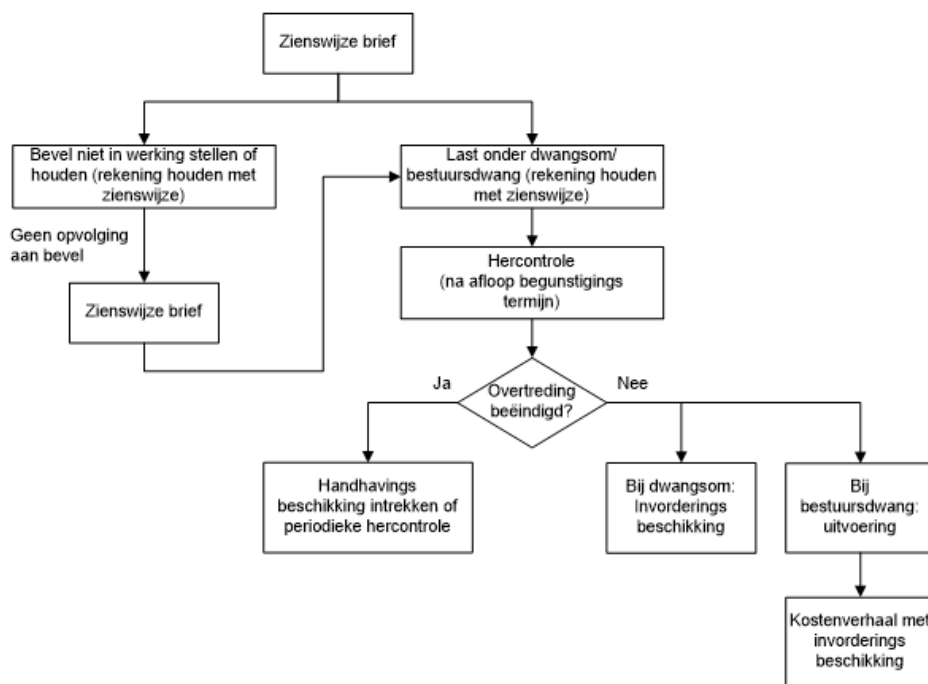
Schema reactie 1
