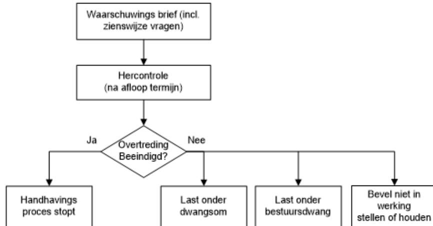
Schema reactie 2
