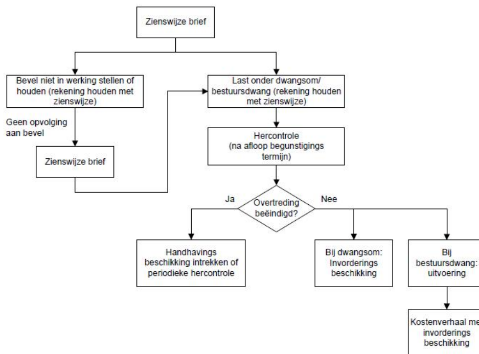
Schema reactie 1
