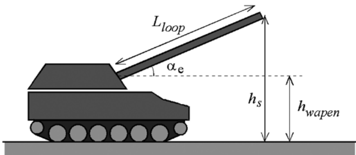
Figuur 4.1: Met de parameters h_{wapen} en L_{loop} kan de hoogte h_s van het bronpunt van de mondingsknaal berekend worden voor een gegeven elevatiehoek \alpha_e . In deze afbeelding valt het bronpunt samen met de vuurmond, maar in het algemeen kan het bronpunt op enige afstand van de vuurmond liggen. L_{loop} is dan langer dan de feitelijke lengte van de loop (zie § 4.5.1).
